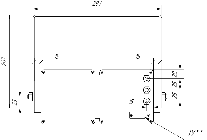
Вид сзади
