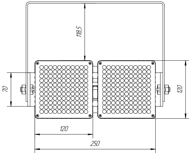
Вид сверху
