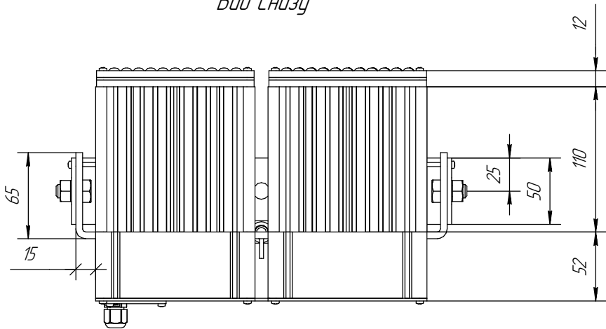
Вид снизу
