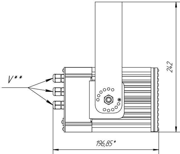
Вид слева
